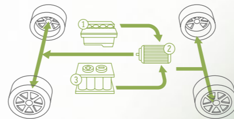
ABB. 3: HYBRIDBETRIEB Je nach Bedarf kommen Elektromotoren und Verbrennungsmotor sowohl bei Stadtfahrten als auch bei Überlandfahrten gemeinsam zum Einsatz.
